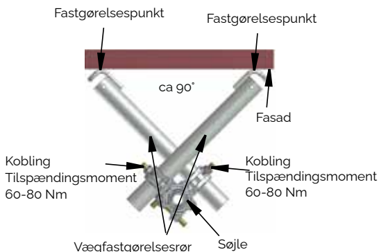
Staging med momenthegn SKRD og forankring
